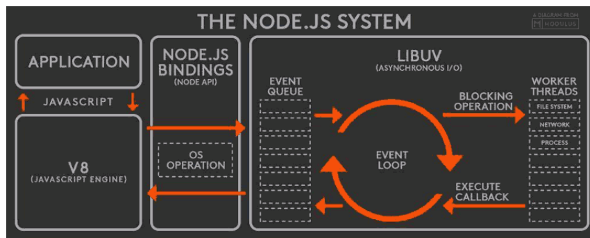
Σχήμα 2.9: Η αρχή λειτουργίας του συστήματος Node.js (Πηγή: [48])
