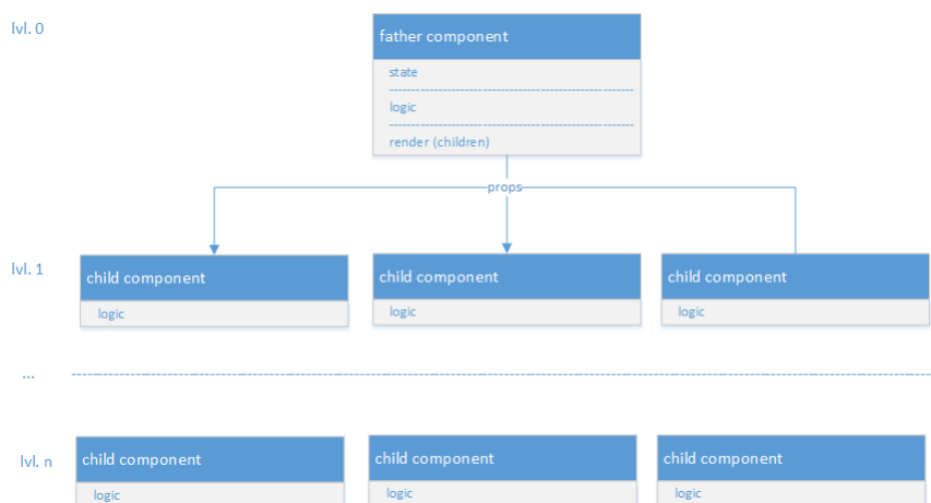
Σχήμα 4.2: Επικοινωνία μεταξύ πατέρα-παιδιών.
