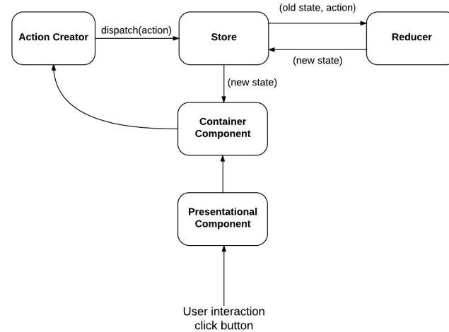
Σχήμα 5.2: Δομή React Redux εντός της εφαρμογής.
