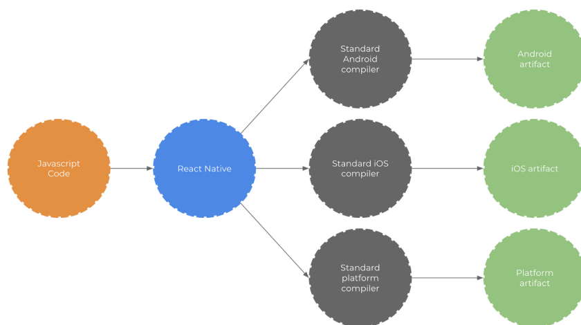
Σχήμα 2.8: Η React Native χρησιμοποιεί τα ίδια native UIs, όπως η Java για Andorid και η Swift για iOS
